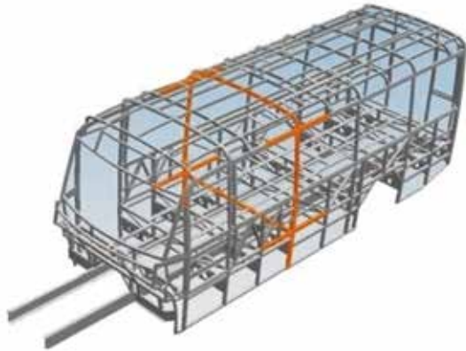
3H High-strength Body (고강도 바디)
