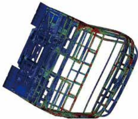
Roll-over Frame Safety (전복보호 구조물)
